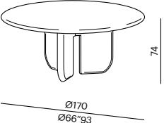
tavolo - table 170R-TP
