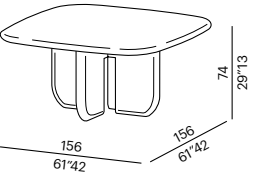
tavolo - table 155-TP
